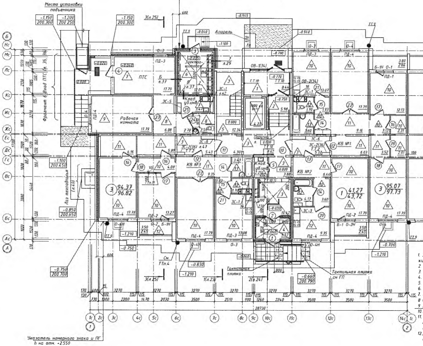
Экспликация отверстий 1-го этажа
